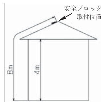
図1. 設置に必要な高さについて
